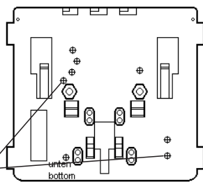
Porte-appareil pour fixation au mur et sur grillage
