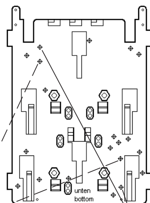
Porte-appareil pour fixation au mur et sur grillage
