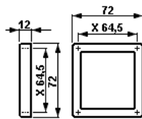
Messinstrumentenvorsatz AM/VM72
